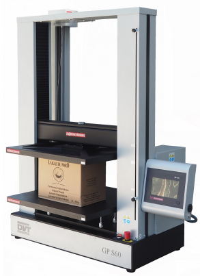
DVT GP D S60 N - TESTEUR DE RESISTANCE A L'ECRASEMENT POUR BOITES
